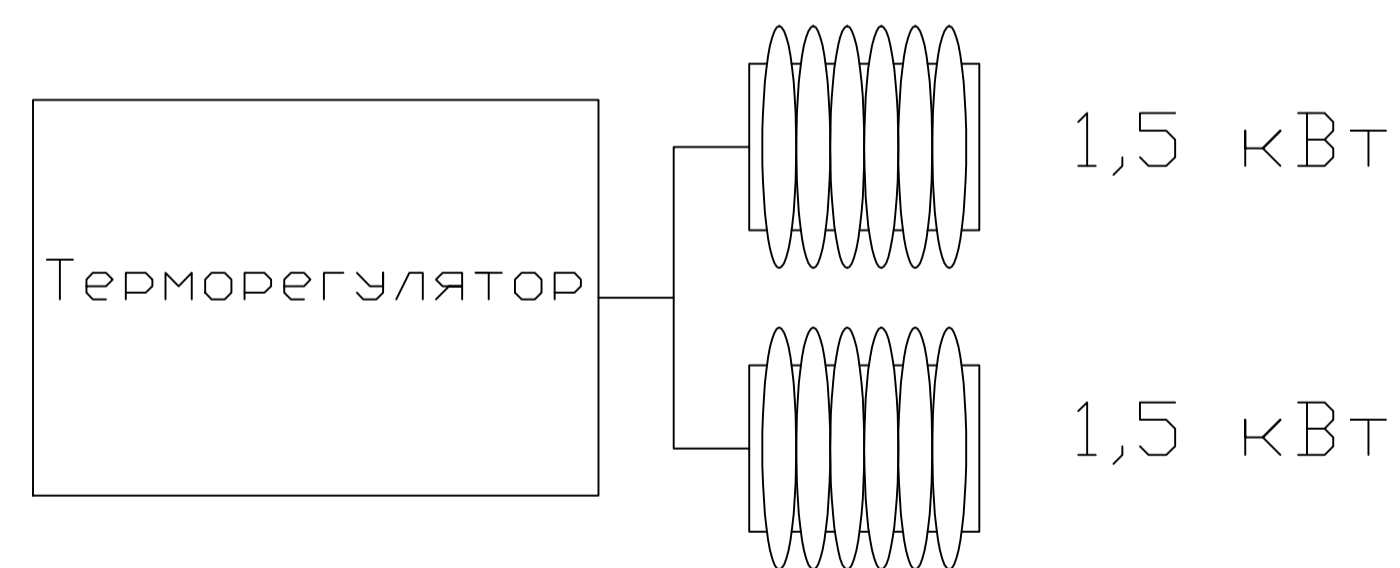
Масляний радіатор
